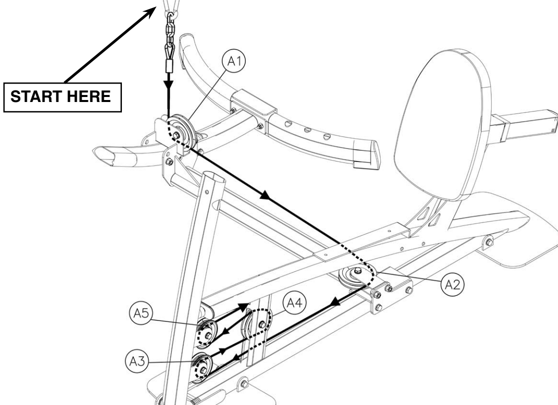
Diagram 2 (pulley installation)
