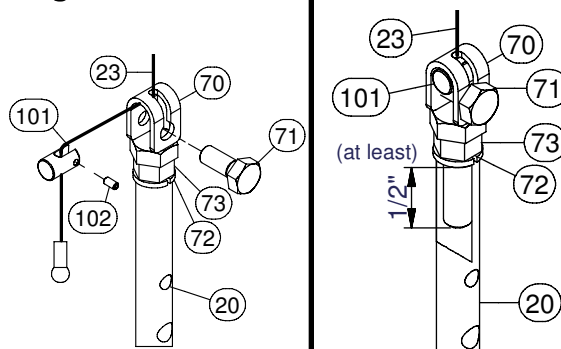
Diagram 1A
